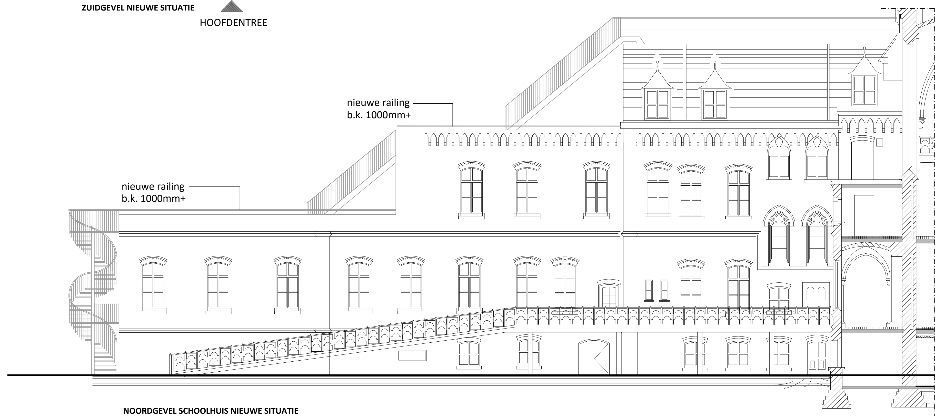
NOORDGEVEL SCHOOLHUIS NIEUWE SITUATIE
