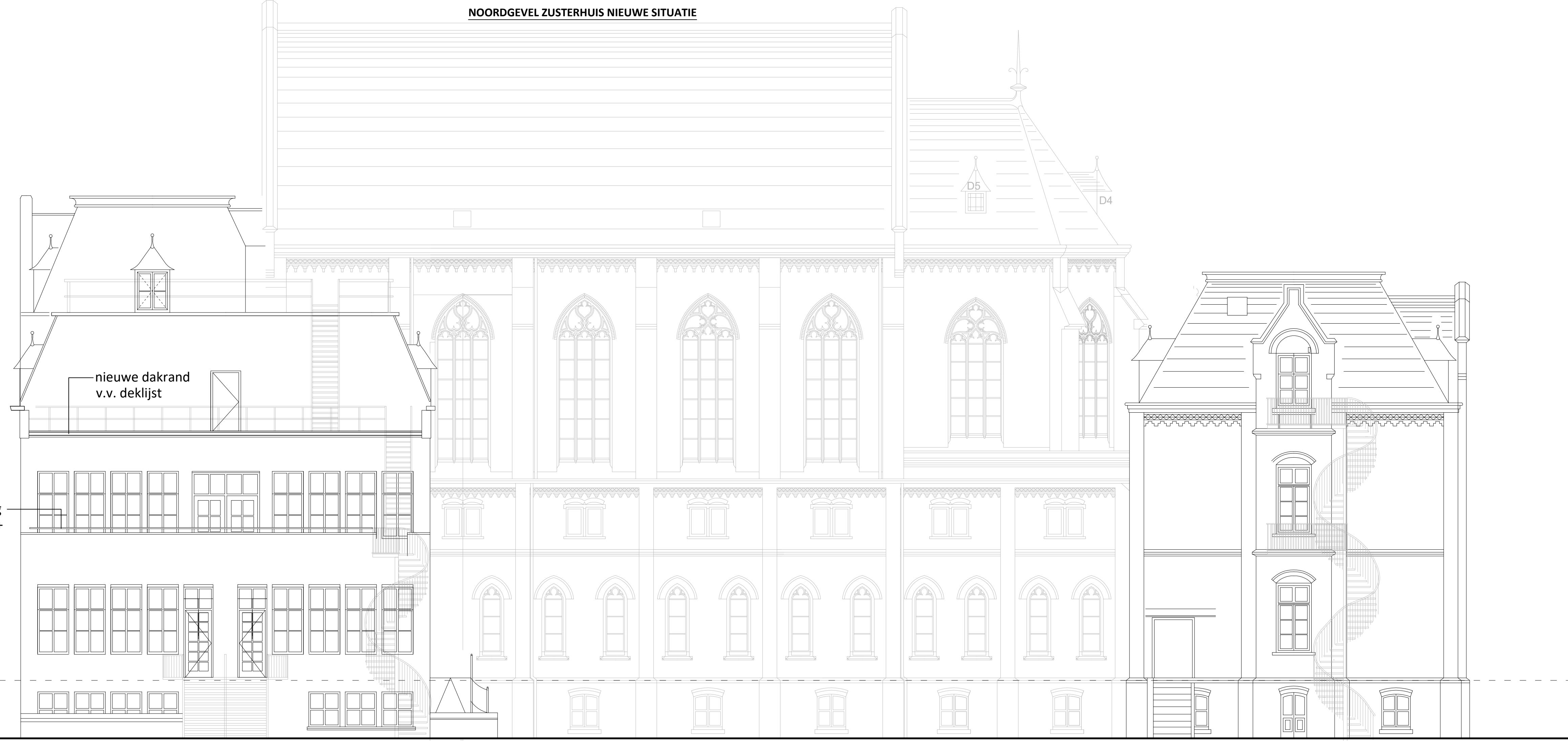
OOSTGEVEL NIEUWE SITUATIE
