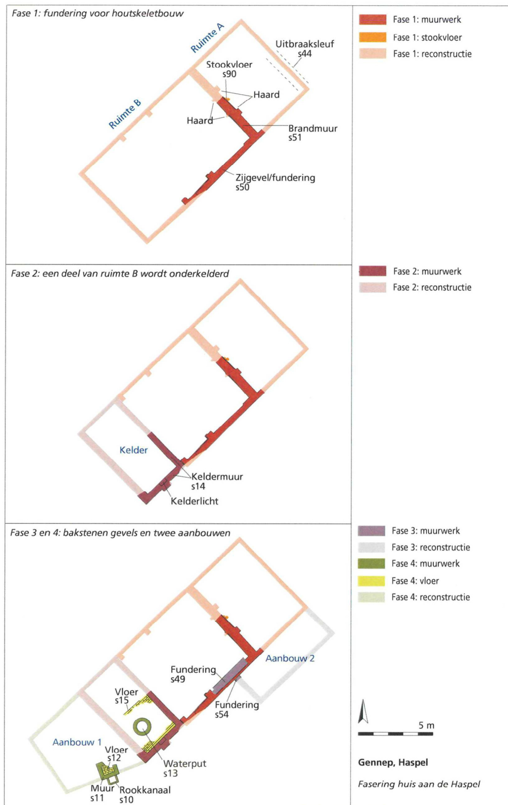
Afb. 3.23 Bouwfases pand.
