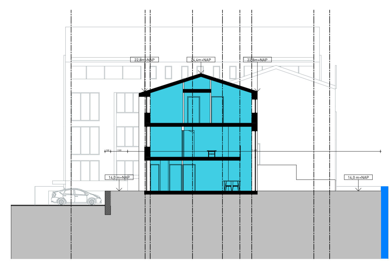
DOORSNEDE A
