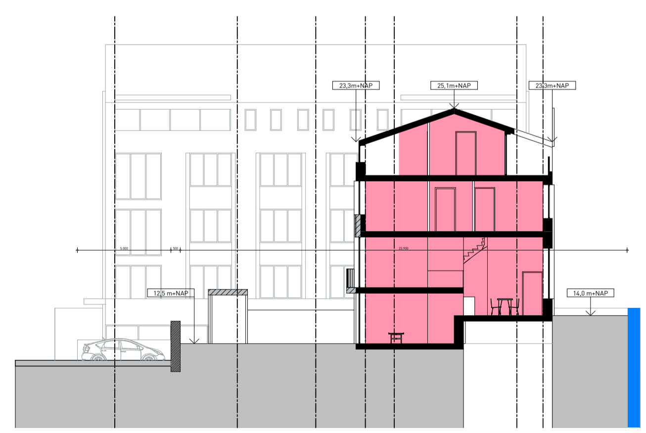
DOORSNEDE B
