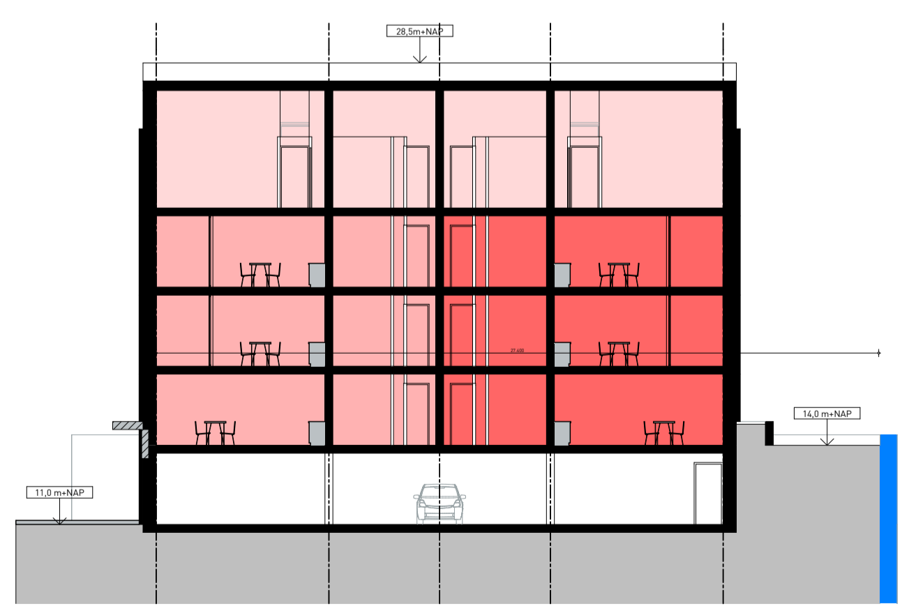
DOORSNEDE C
