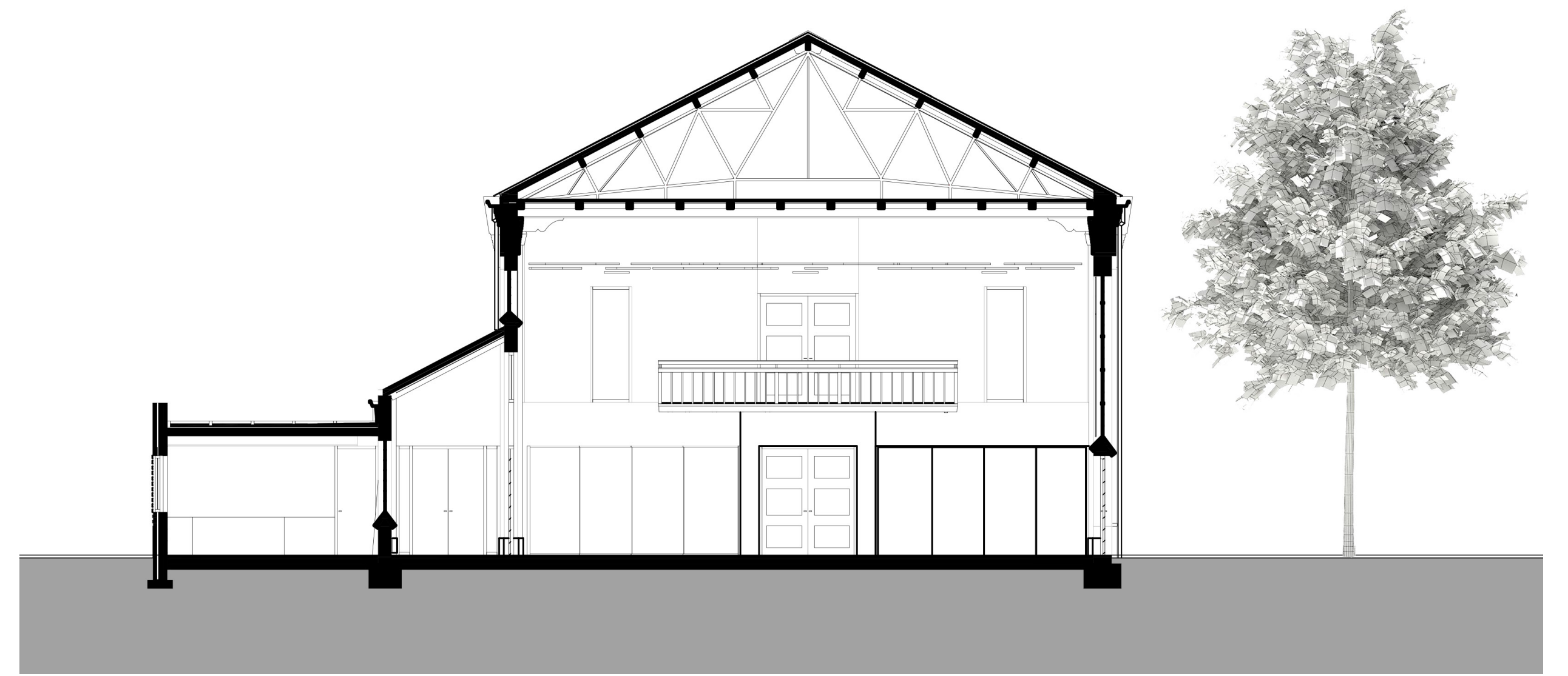
DOORSNEDE A-A
