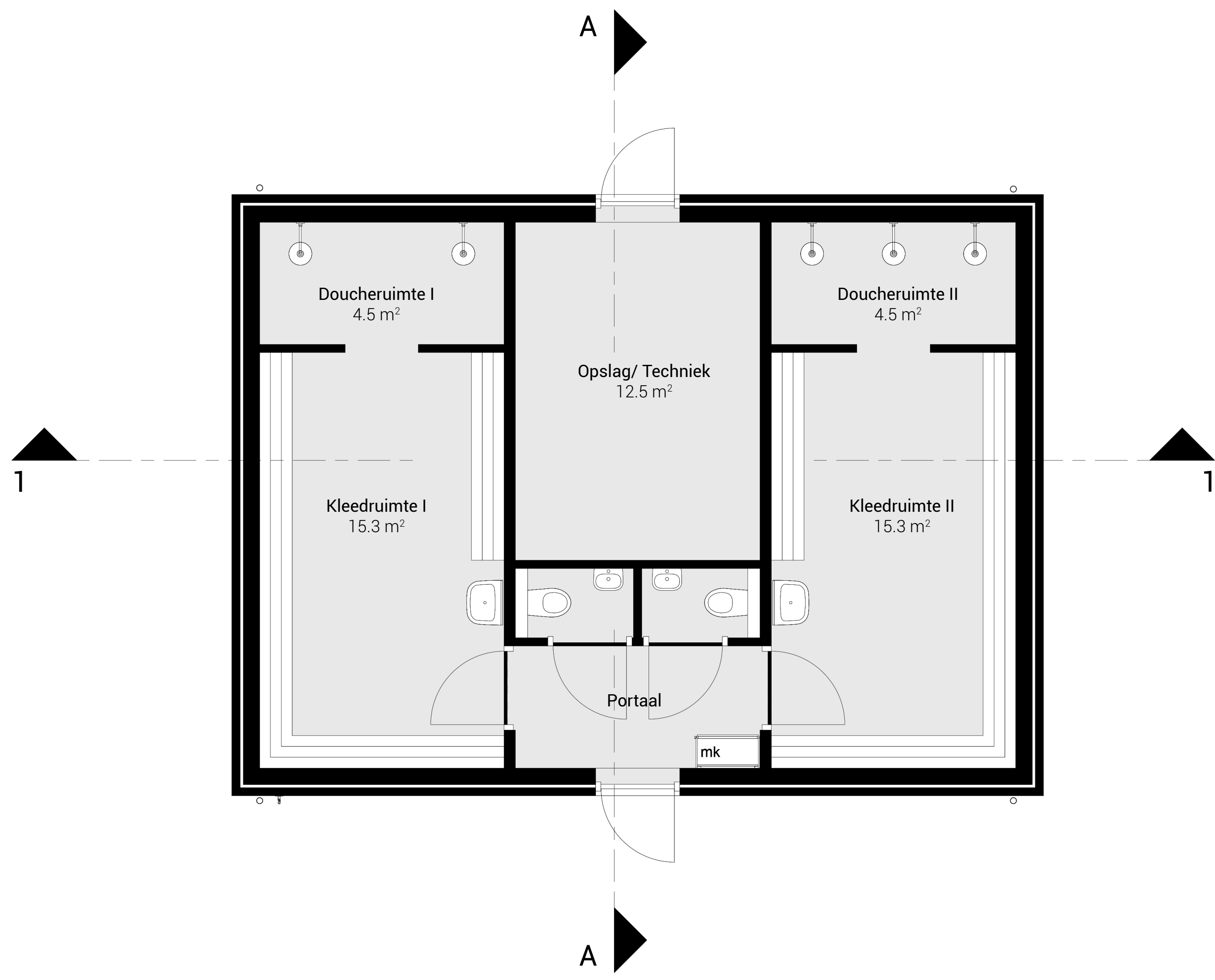
BEGANE GROND
