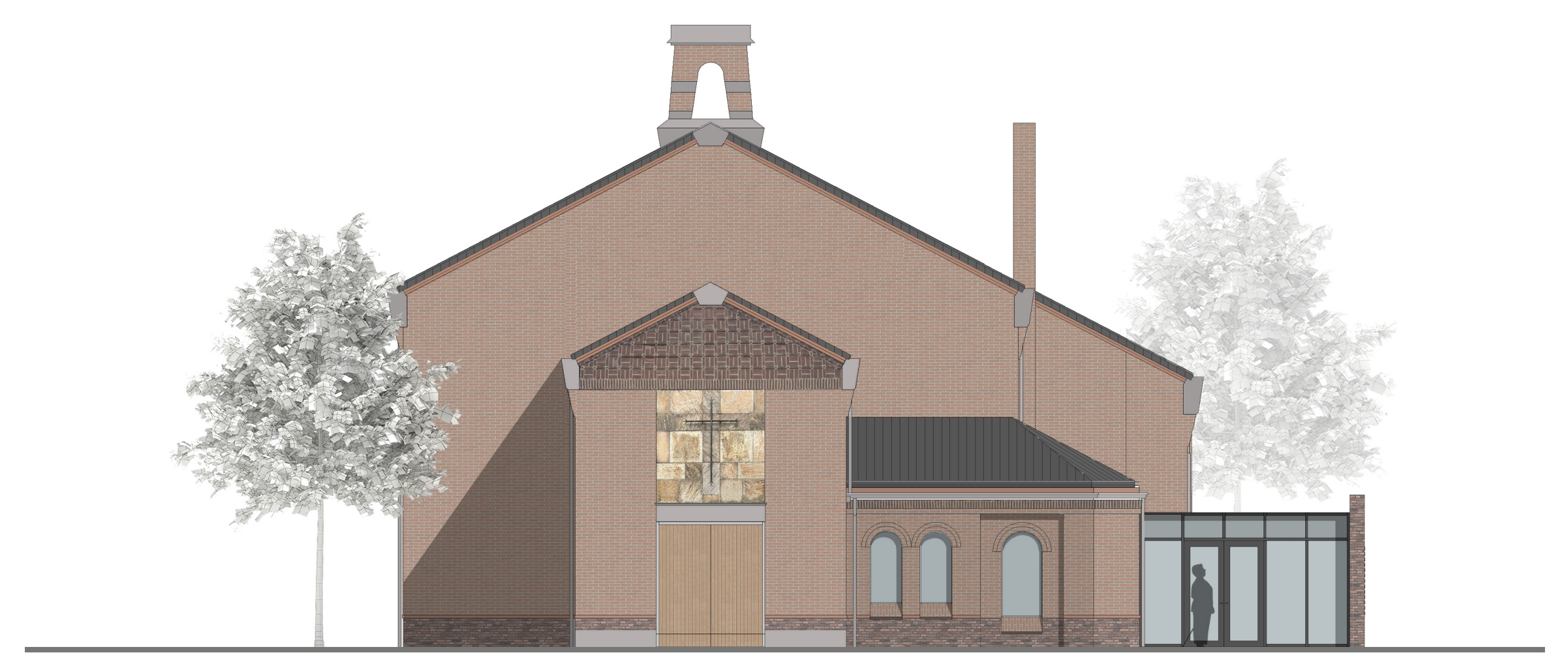
RECHTER ZIJGEVEL
