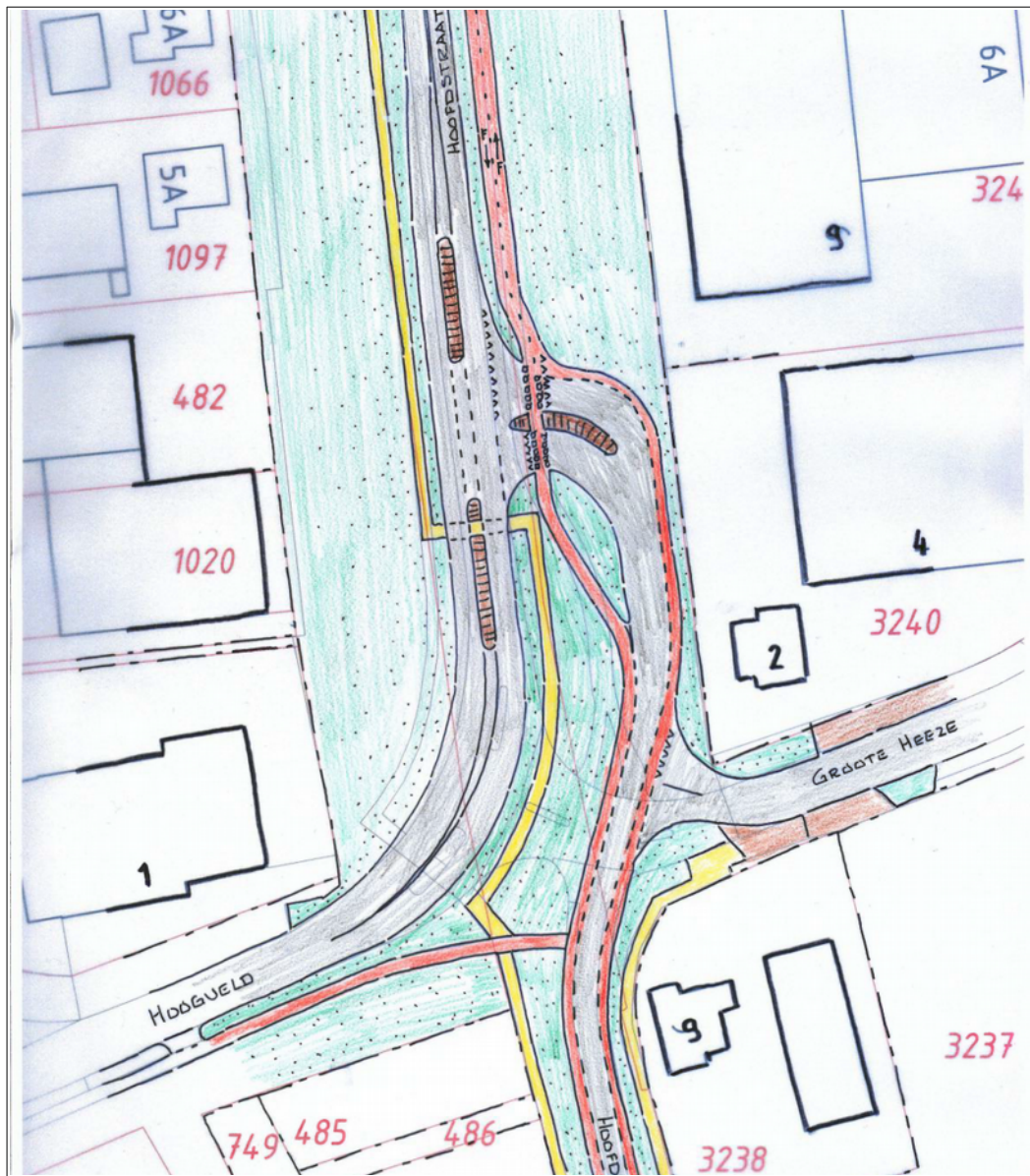
f2.2 Herinrichting kruispunt Hoofdstraat/Hoogveld/De Grootte Heeze.
